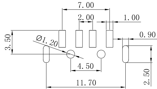
91-US01-XXX PCB LAYOUT
