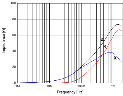
HB-1H1608-300J
