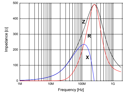
HB-1M3216-301J
