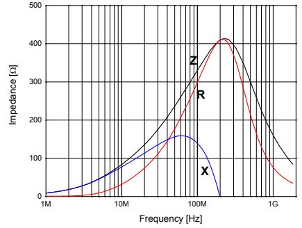
HB-1T2012-331J
