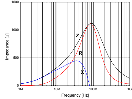
HB-1T2012-102J
