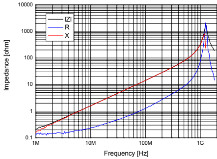
HB-1Y1608-150J
