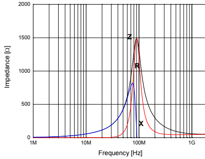
HH-1B4532-132J
